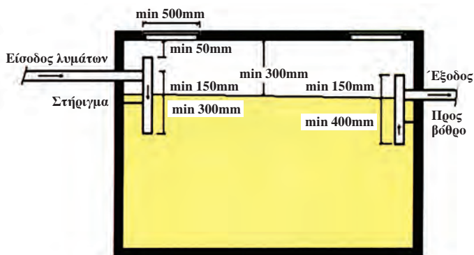
ΣΧ.5.2.1.α Μονοθάλαμος στεγανός βόθρος.
