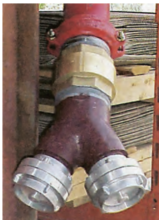
ΣΧ. 10.2.2.α Δίδυμο πυροσβεστικό υδροστόμιο, σε βιομηχανία.
