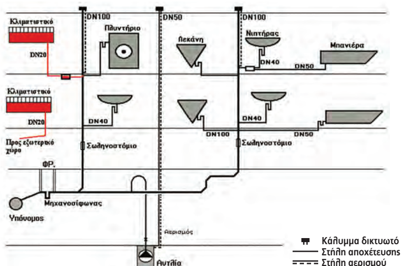
ΣΧ. 3.9.γ Κατακόρυφο σχέδιο αποχέτευσης με είδη υγιεινής και κλιματιστικά. Οι κλιματιστικές συσκευές αποχέτευονται είτε σε σιφώνια δαπέδου, που γεμίζουν συνεχώς με νερό, είτε έξω στο περιβάλλον. Δε συνδέονται ποτέ απ' ευθείας σε στήλες αποχέτευσης.
