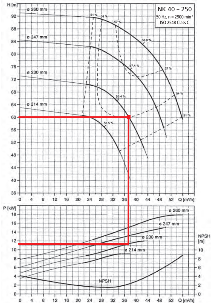
ΣΧ.9.1.4.α Τυπικές καμπύλες λειτουργίας φυγοκεντρικής αντλίας. Η ίδια αντλία μπορεί να κατασκευαστεί με τέσσερις φτερωτές διαμέτρων 214mm, 230mm, 247mm και 260mm. Οι αντίστοιχες καμπύλες λειτουργίας δείχνουν τις παροχές της αντλίας για κάθε μονομετρικό. Π.χ. για τη φτερωτή 230mm, όταν το μονομετρικό είναι 60m, τότε η παροχή της αντλίας είναι 37,5m 3 /h και η απαιτούμενη ισχύς του ηλεκτροκινητήρα είναι 11 kW. Με τη φτερωτή αυτή η παροχή μπορεί να φθάσει τα 44m 3 /h, αλλά σε μονομετρικό 47m.
