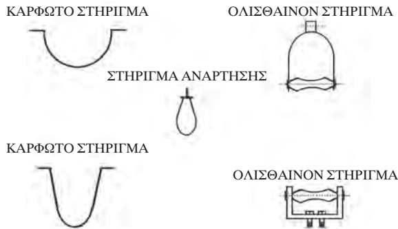
ΣΧ.8.2.4.α Είδη στηριγμάτων δικτύων.
