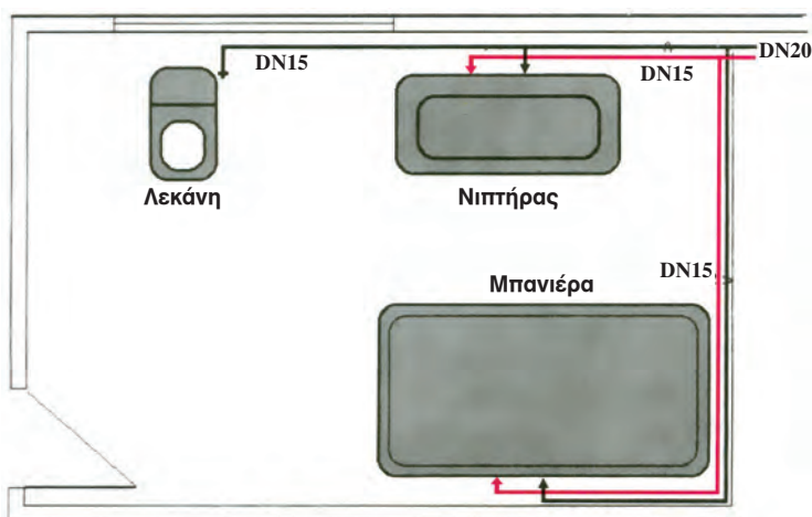
ΣΧ. 2.15.2.α Υδροδότηση μπάνιου
