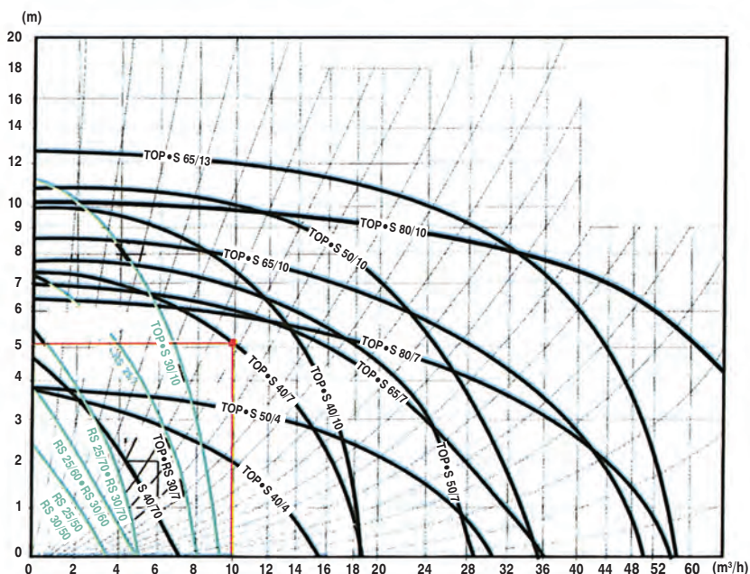
ΣΧ.9.3.β Τυπικές καμπύλες λειτουργίας κυκλοφορητών. Αν θέλουμε έναν κυκλοφορητή με σημείο λειτουργίας: παροχή 10 \text{ m}^3/\text{h} και μανομετρικό 5\text{m} , με βάση τις καμπύλες αυτές θα επιλέξουμε τον τύπο TOP S40/7 .
