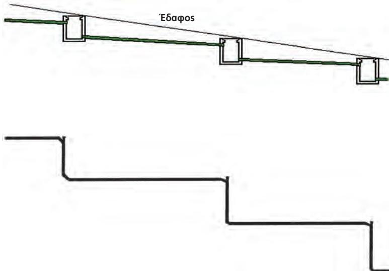
ΣΧ. 3.14.5.β Φρεάτια πτώσης στάθμης και κατακόρυφη μετατόπιση αγωγών αποχέτευσης.
