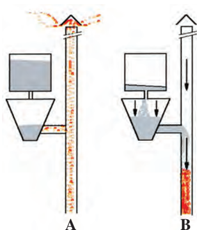
ΣΧ. 3.6.3.α Λειτουργία στήλης αποχέτευσης - αερισμού
