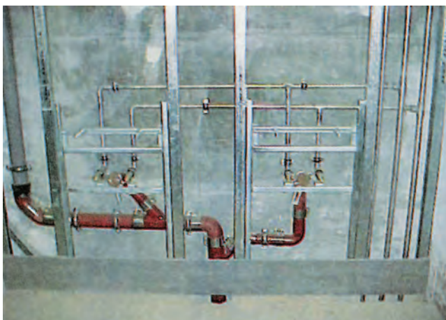
ΦΩΤ. 2.14.α Υδραυλική εγκατάσταση με διακλάδωση σωλήνων. Οι δυο κύριες γραμμές, ζεστού και κρύου νερού, τροφοδοτούν με διακλαδώσεις τους δυο νιπτήρες. Χρησιμοποιήθηκαν γαλβανισμένοι σιδηροσωλήνες. Οι διακλαδώσεις και οι αλλαγές διεύθυνσης του δικτύου έγιναν με ειδικά εξαρτήματα (μούφες, ταφ, γωνίες).
