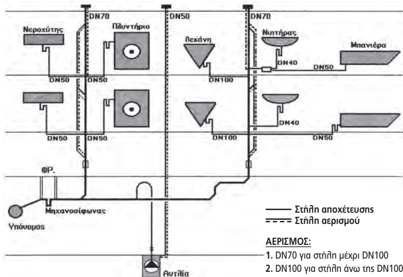
ΣΧ. 3.6.6.γ Κατακόρυφο διάγραμμα αποχέτευσης με “Πλήρη αερισμό”. Είναι η πλέον ολοκληρωμένη μέθοδος αερισμού αλλά και η πιο δύσκολη και δαπανηρή.
