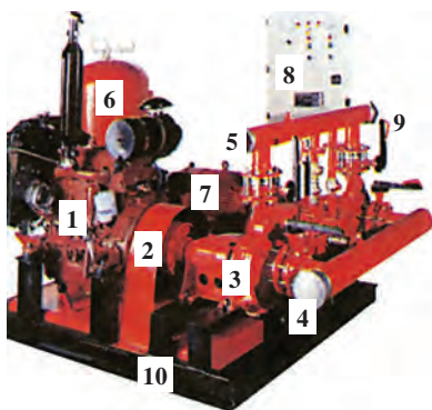
ΣΧ. 10.2.4.α Πλήρες πυροσβεστικό συγκρότημα. Διακρίνονται: η πετρελαιοκίνητη αντλία (1), ο συμπλέκτης πετρελαιοκινήτρια - αντλίας (2), η αντλία (3), ο συλλέκτης αναρρόφησης νερού (4), ο συλλέκτης διανομής νερού (5), το πιεστικό δοχείο (6), ο ηλεκτροκινήτριας της δεύτερης αντλίας (7), ο πίνακας αυτοματισμών (8), οι υδραυλικοί διακόπτες (9) και η ενιαία βάση στήριξης (10).
