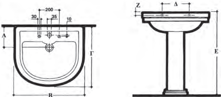
ΣΧ.7.4.α Νιπτήρας και βασικές του διαστάσεις.
